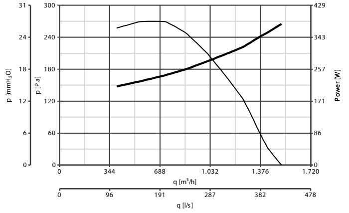
C 35/4 ME
