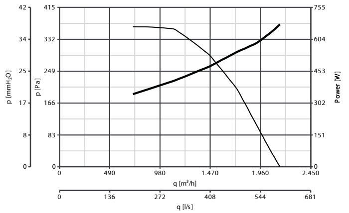
C 37/4 ME
