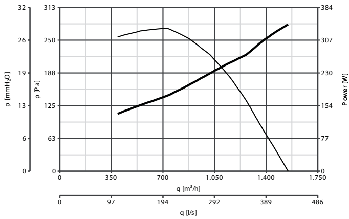
C 35/4 TE
