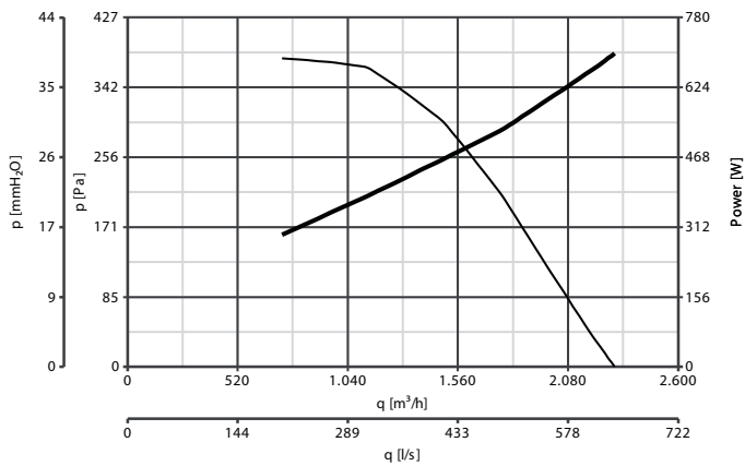
C 37/4 TE
