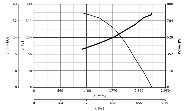
C 40/4 ME
