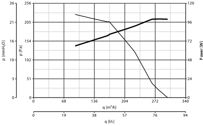
C 10/2 M
