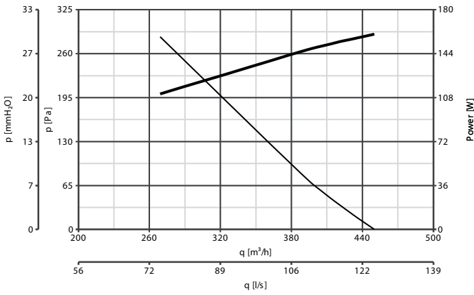
C 15/2 M
